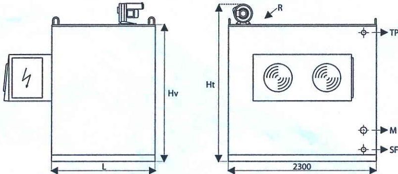
TIPO A / TYPE A: Vasca con gruppo frigo premontato / Tank with premounted cooling unit
