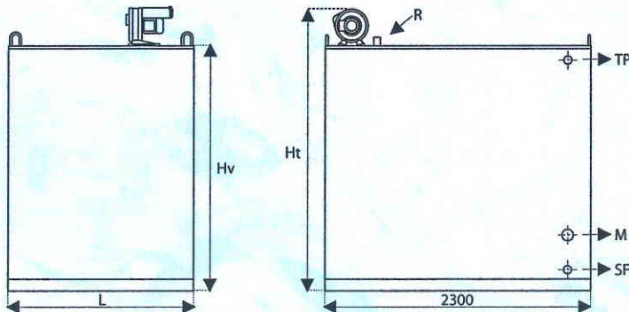
TIPO B / TYPE B: Vasca con gruppo frigo separati / Tank with remote cooling unit
