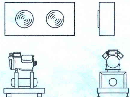
TIPO C / TYPE C: Vasca, unità e condensatore separati / Tank with remote condensing unit and remote condenser
