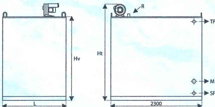
TIPO C / TYPE C: Vasca, unità e condensatore separati / Tank with remote condensing unit and remote condenser
